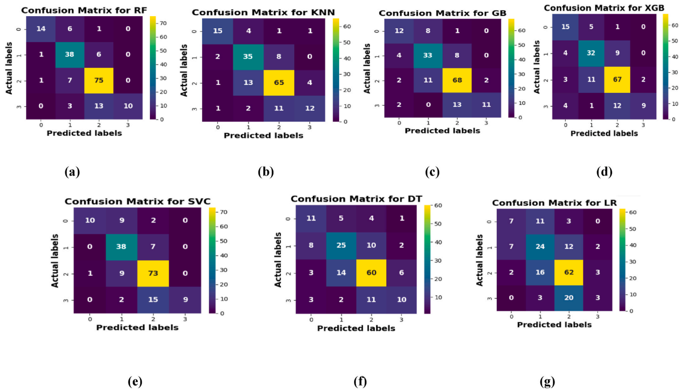
Fig. 7. 4x4 Confusion Matrix for ML classifier ((a) RF (b) KNN (c) GB (d) XGB (e) SVC (f) DT (g) LR) After Applying Scaling Techniques.
